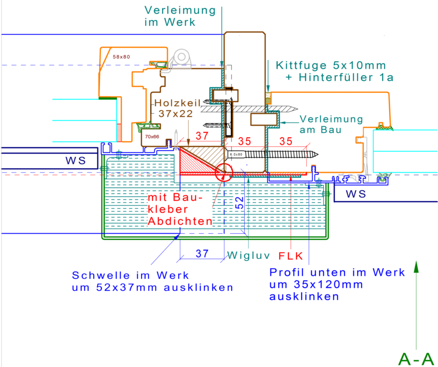
Ansicht A-A
