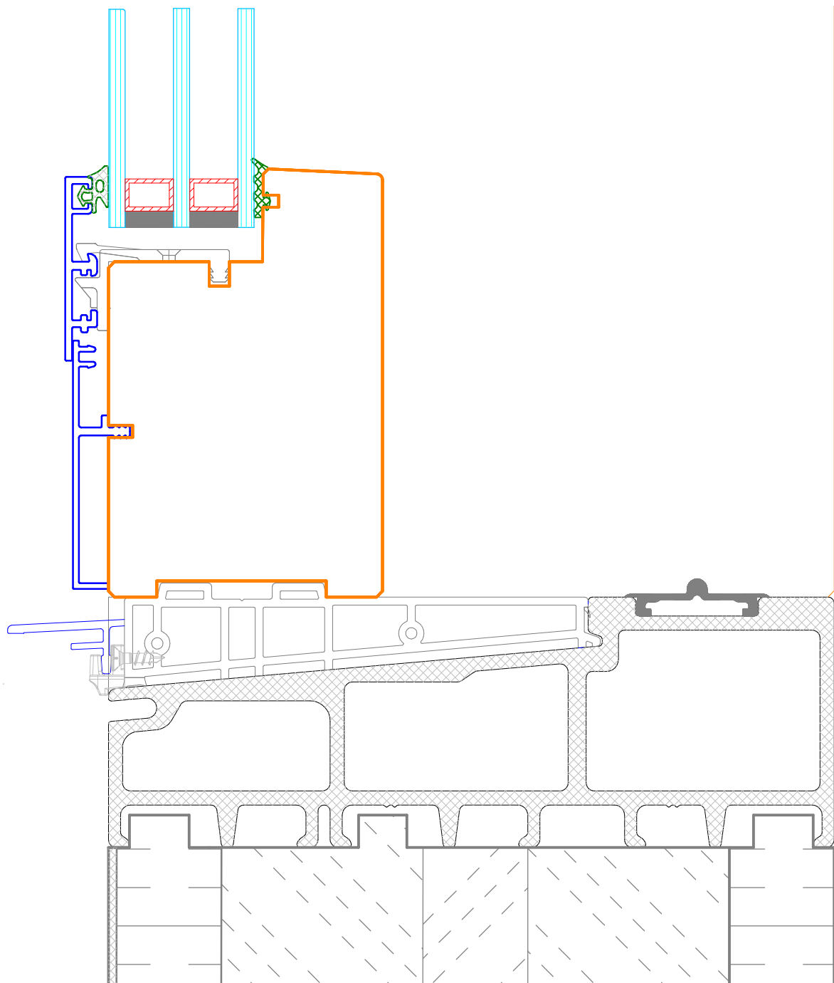
Variante mit schwollenlosem Austritt
